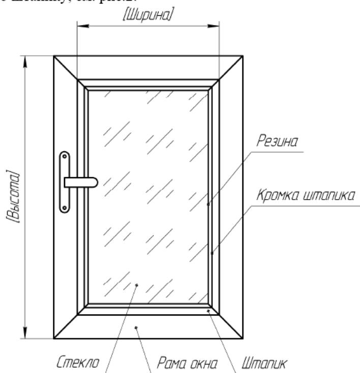
Рис.2. Замер для установки на раму окна
